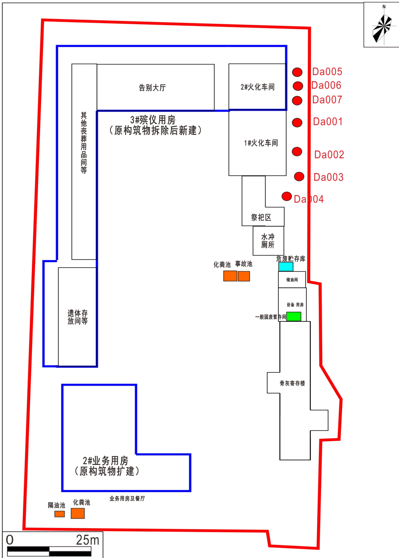
附图 6 建设项目平面布置图
