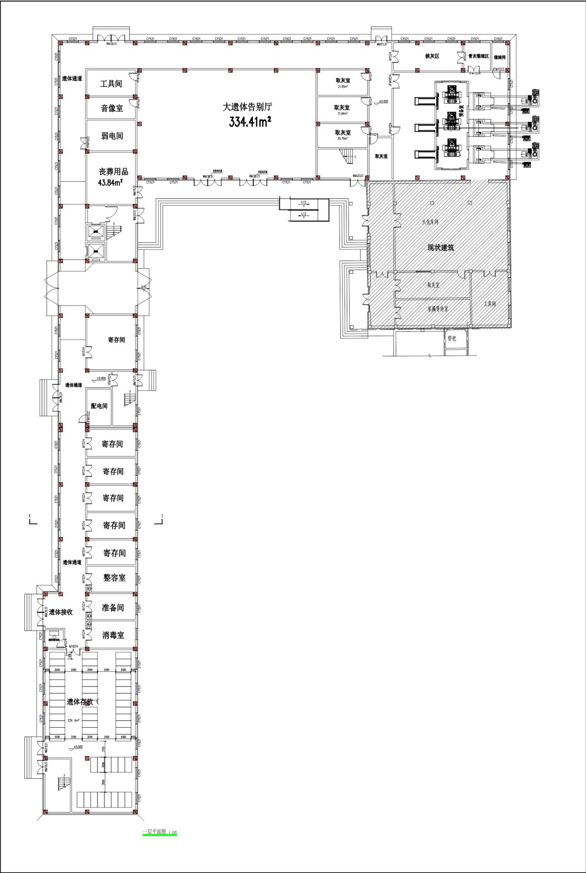
附图9 3#殡仪用房1层平面布置图
